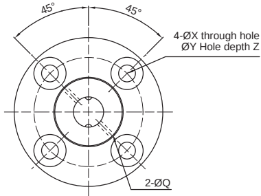
【Two Starts】Type : 06、10、13
