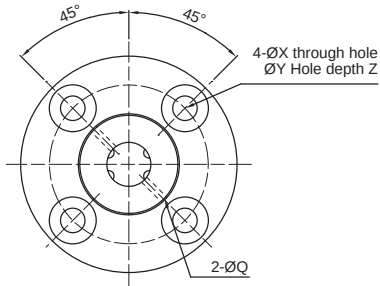
【Four Starts】Type : 40、50
