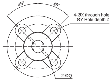
【Four Starts】Type : 25、30
