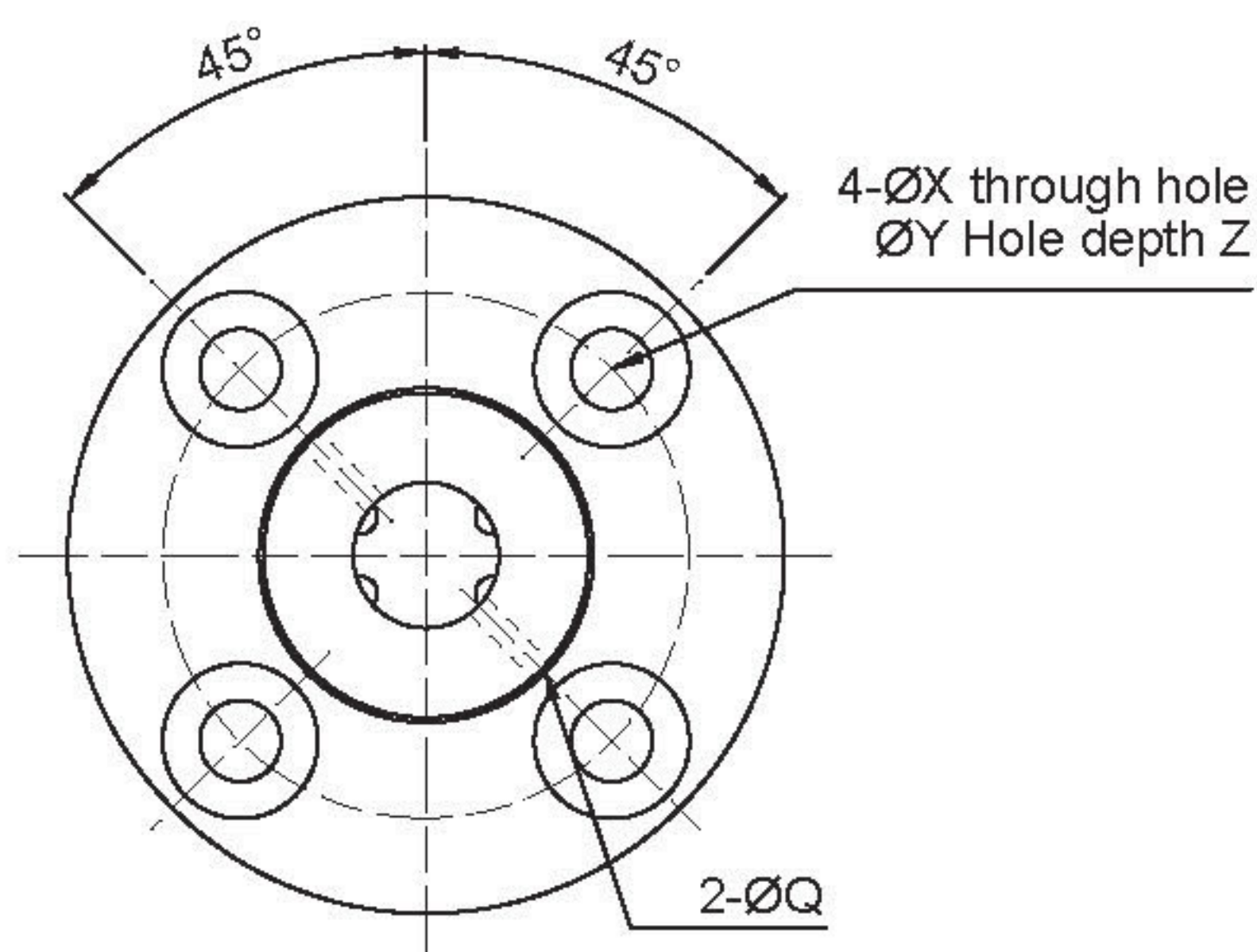
【Four Starts】Type : 40、50
