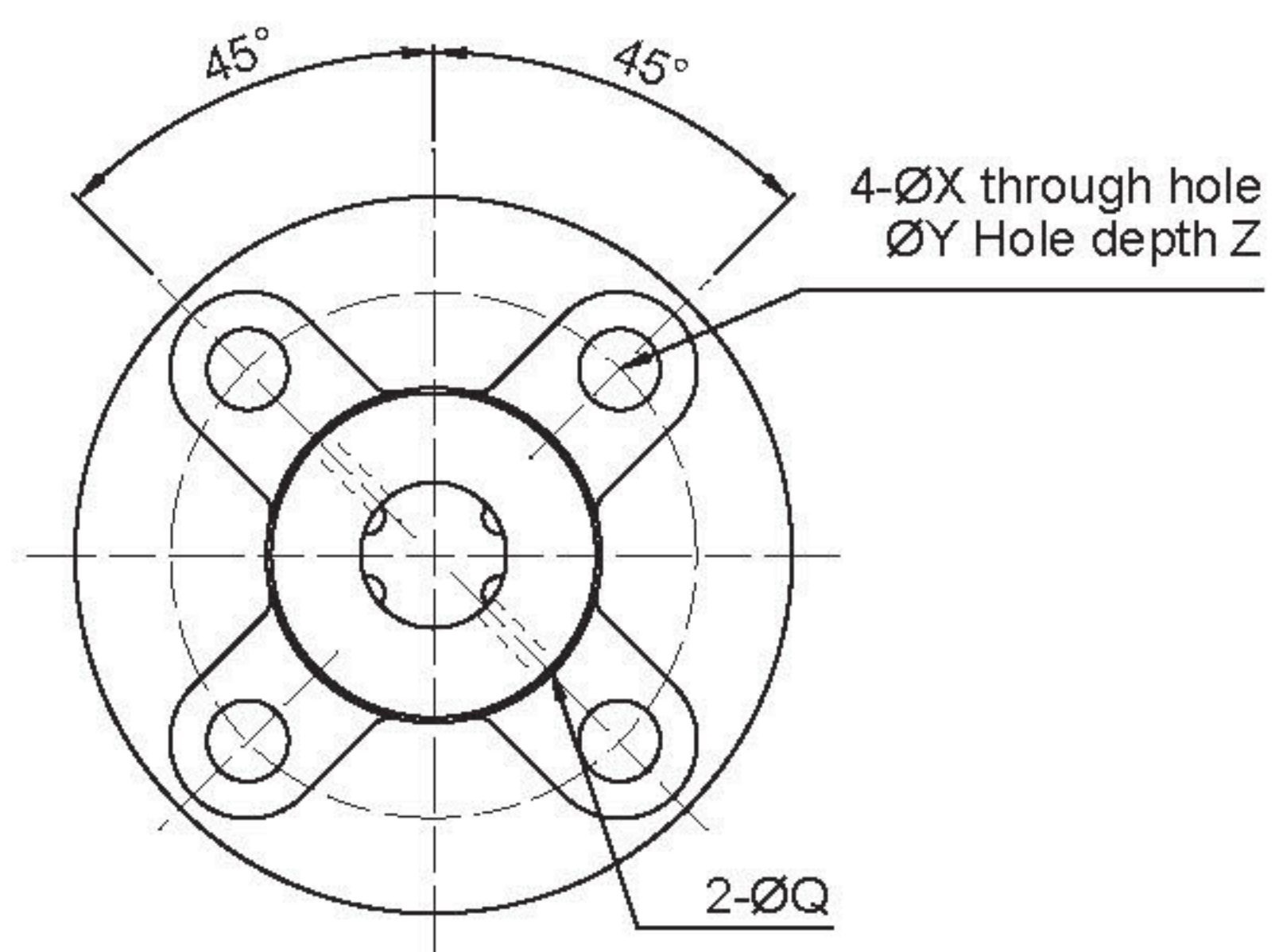
【Four Starts】Type : 25、30
