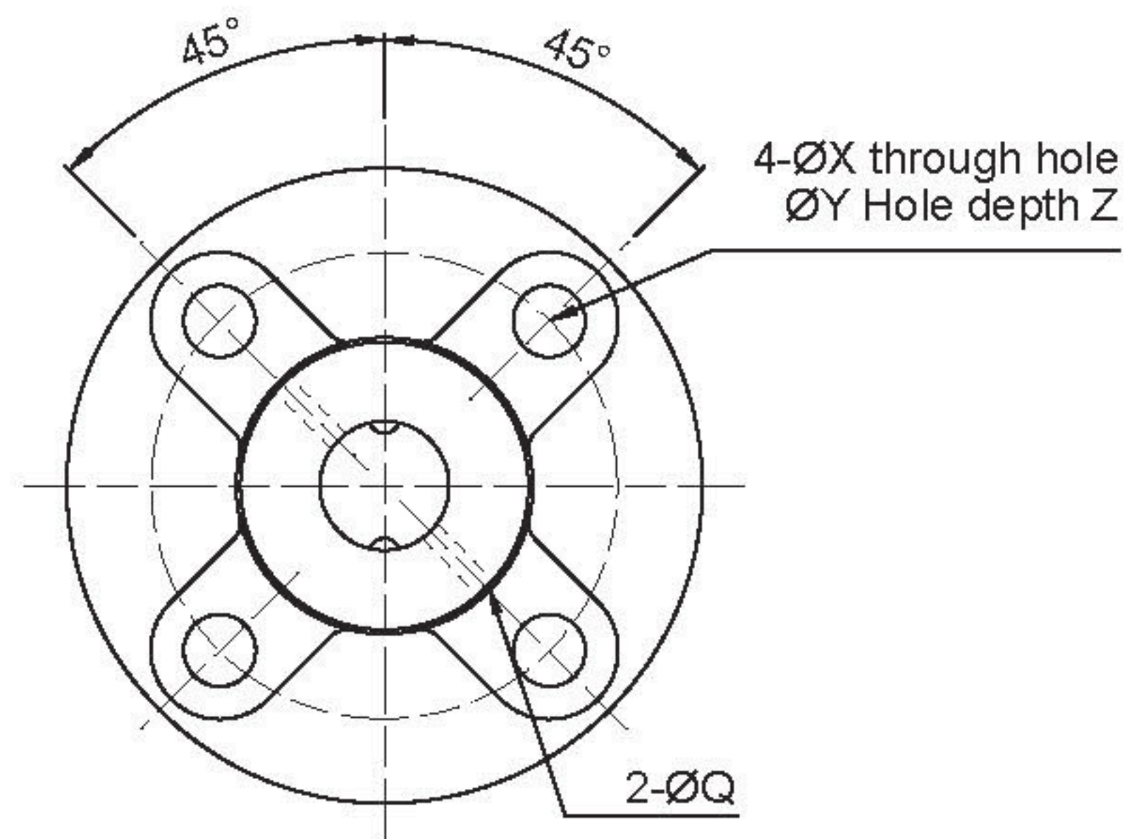
【Two Starts】Type : 08、16、20
