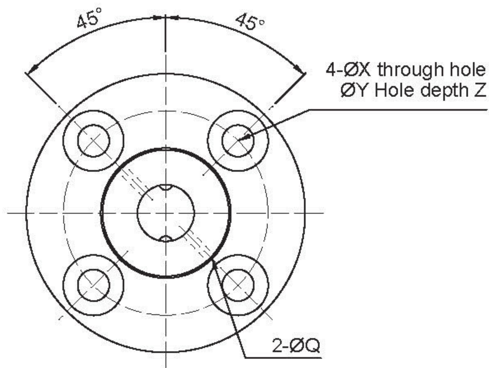
【Two Starts】Type : 06、10、13
